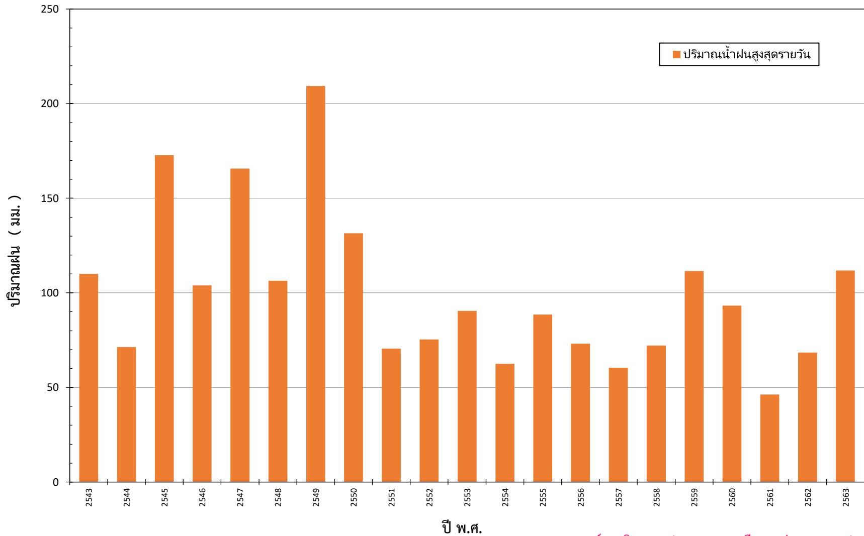
กราฟแสดงปริมาณฝนสูงสุดรายวัน ปีพ.ศ. 2543 - 2563 สถานีน้ำฝน ศอช.ภาคเหนือตอนล่าง ( 390220 ) อ.เมือง จ.
